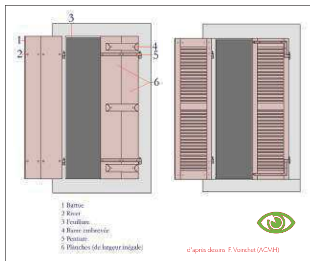
Modèles de fenêtres traditionnelles à conserver et mettre en œuvre.
